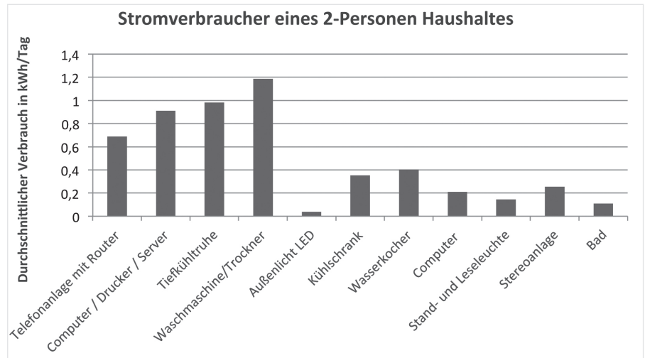
Beispielhafte Auswertung einer Messung von verschiedenen Stromverbrauchern; Quelle: KBN
